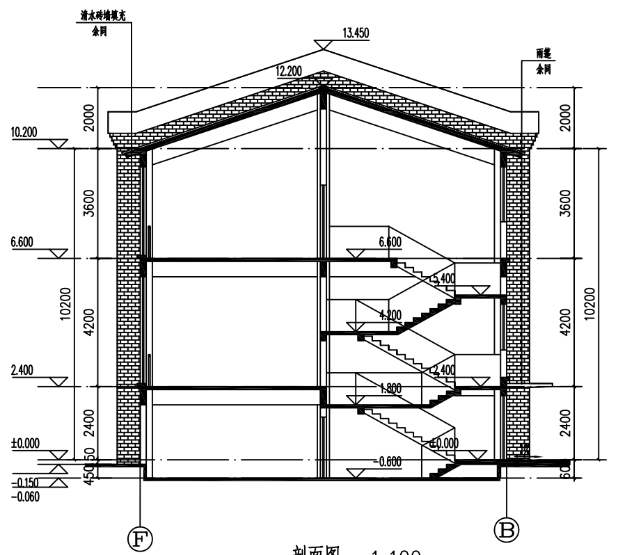
剖面图 1:100
