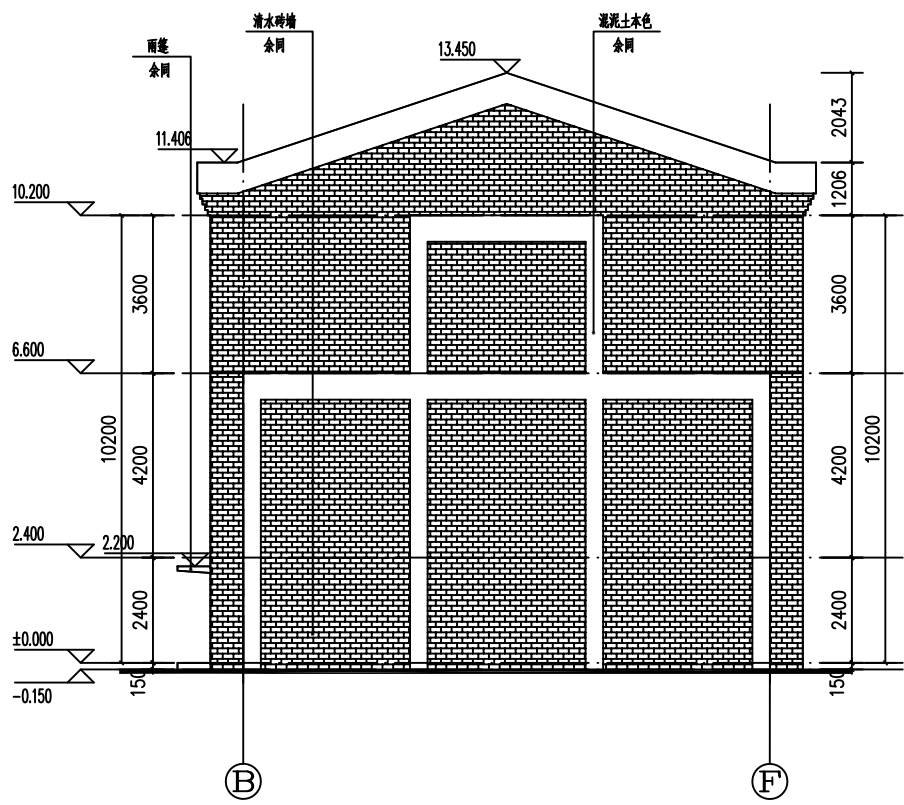
② - ⑥ 立面图 1:100
