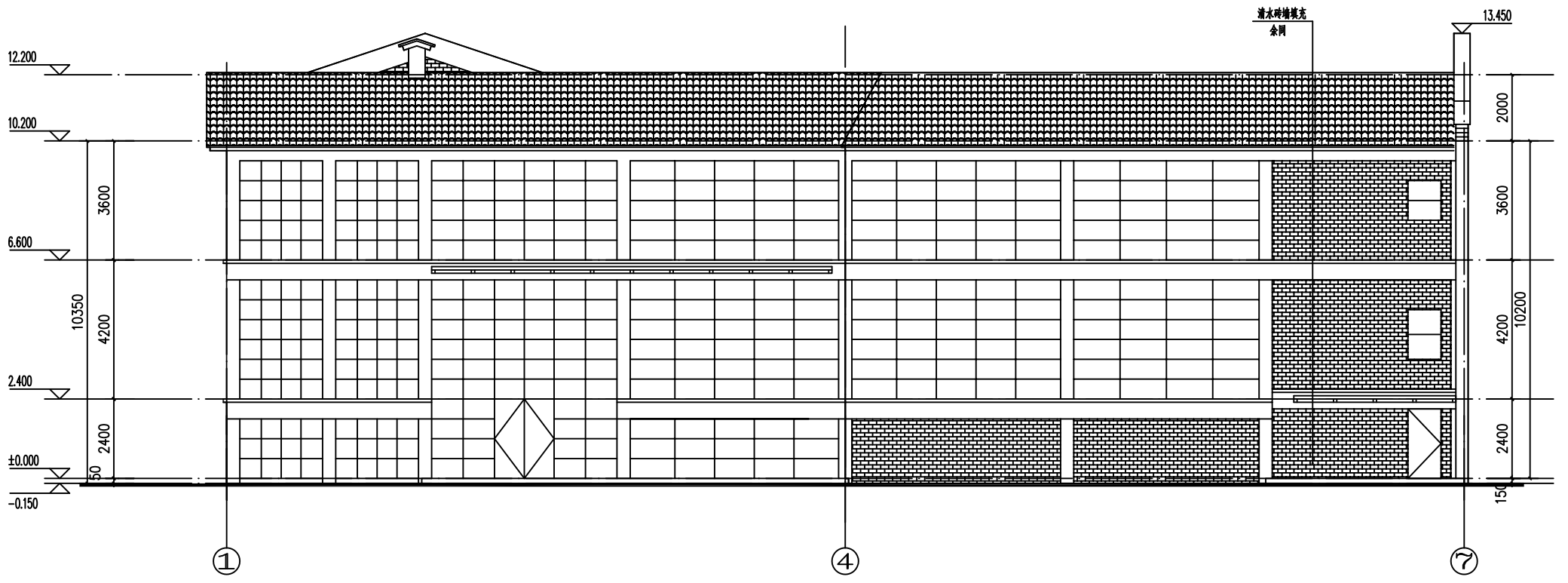
①-⑦ 立面图 1:100
