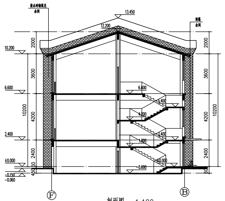
剖面图 1:100
